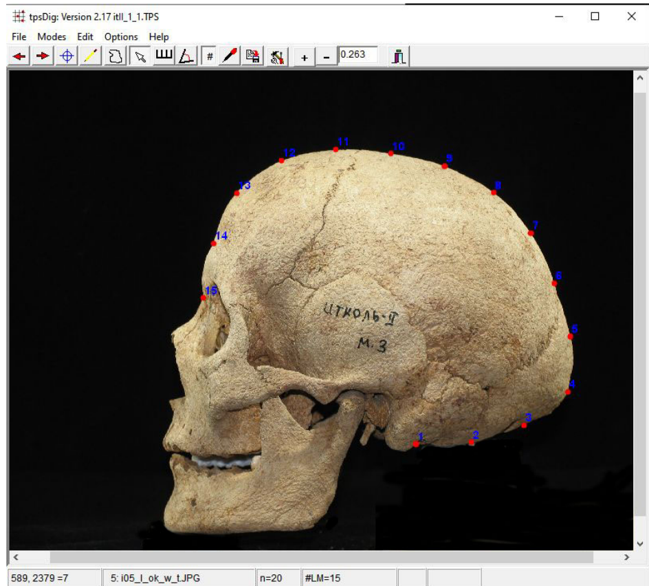
Рис. 2. Точки и полуточки (landmarks и semilandmarks) на сагиттальном контуре черепа (программа из серии TPS)
