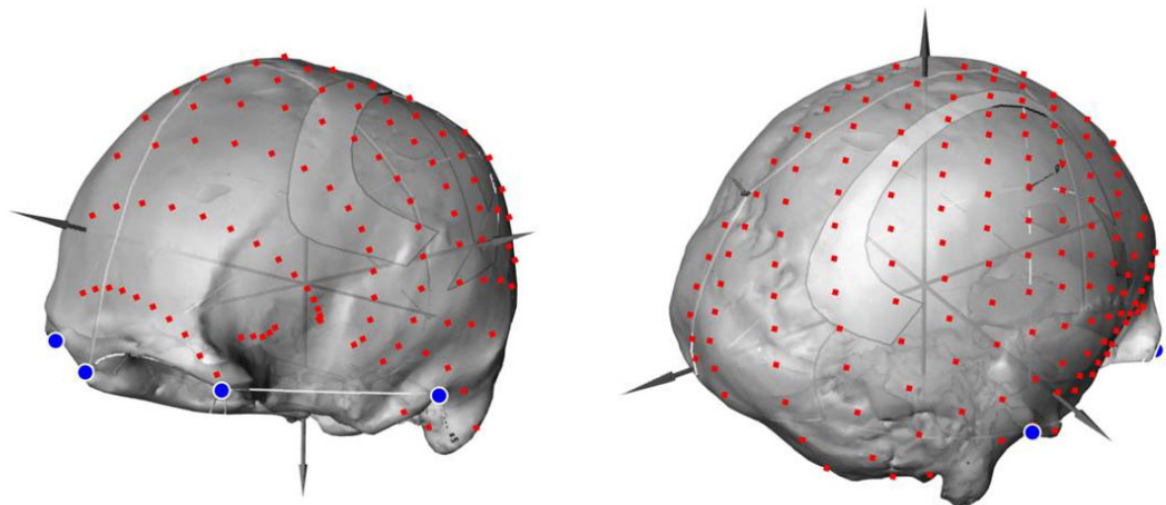
Рис. 3. 3D-модели мозговых частей черепа с расставленными точками (landmarks, синие) и полуточками (semilandmarks, красные)
